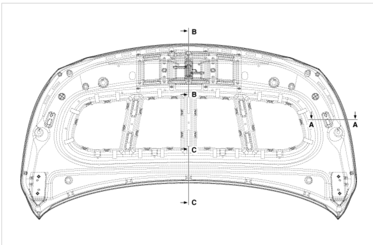
A - A
